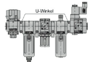
Verbindung Baureihe GZ, GV und GC
