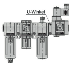
Verbindung Baureihe GV und GC
