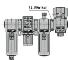
Verbindung Baureihe GZ und GC
