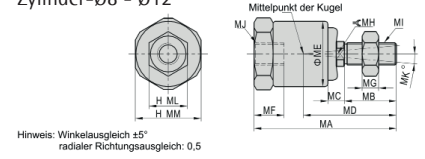
Zylinder-Ø8 - Ø12
