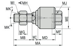
Zylinder-Ø20 - Ø40
